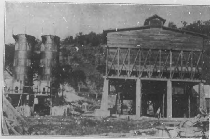
Vista de los depósitos, trituradora y hornos de cal de la "Compañía Calera Cubana" de Siguaney.
